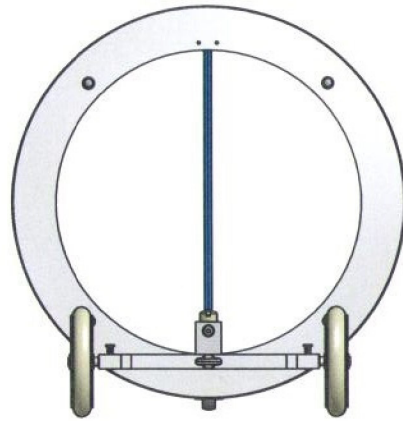
VP700-800 Rohr DN700
